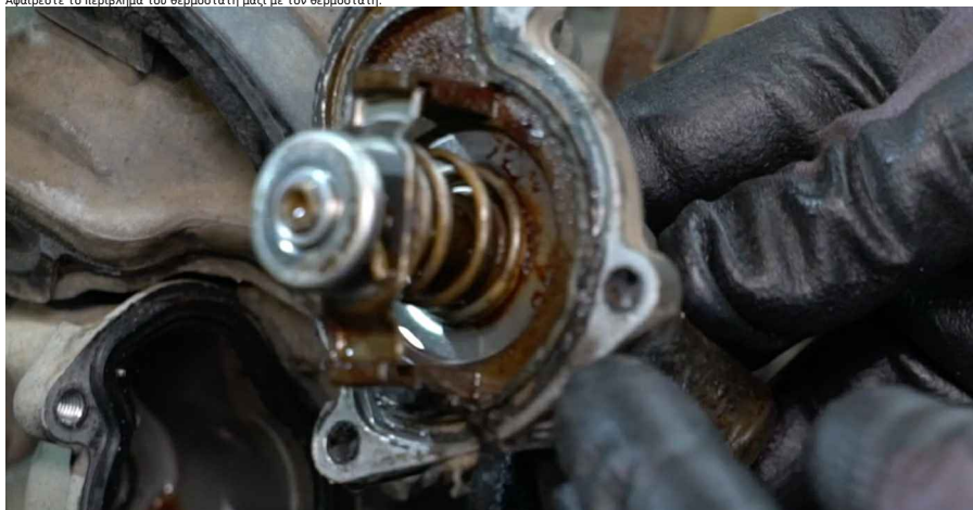
22 Καλύψτε τη βάση στήριξης του περιβλήματος θερμοστάτη με ένα παξι μικροίτων, για να εμποδίσετε την είσοδο σε ακαθαρσίες και ξένα αντικείμενα στο σύστημα.
