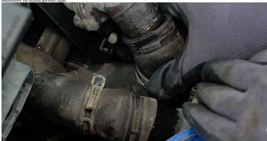
Αντικατάσταση: θερμοστάτης - VAUXHALL ASTRA Mk II Στέισον βάγκον. Το ΑΥΤΟΔΟC συνιστά: • Προσοχή! Το ψυκτικό μπορεί να διαρρέουσι από τις γραμμές ψυκτικού και το περίβλημα του θερμοστάτη.
